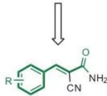
21a-21b
