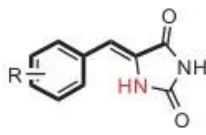
18a (hydatoin)
