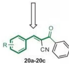
20a-20c
