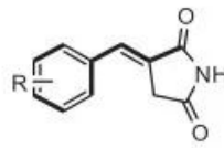
18b (pyrrolidinedione)
