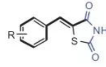
18c ( thiazolidinedione)
